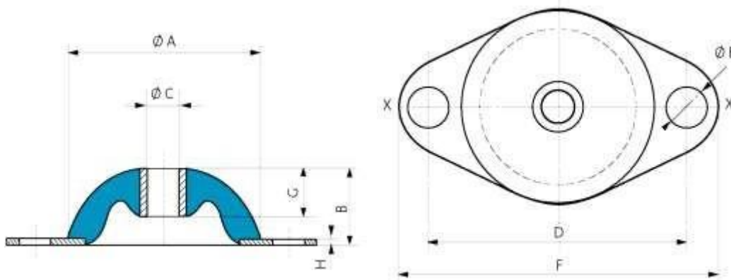
Сечение XX'
