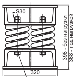
Шпилька монтажного сжатия
